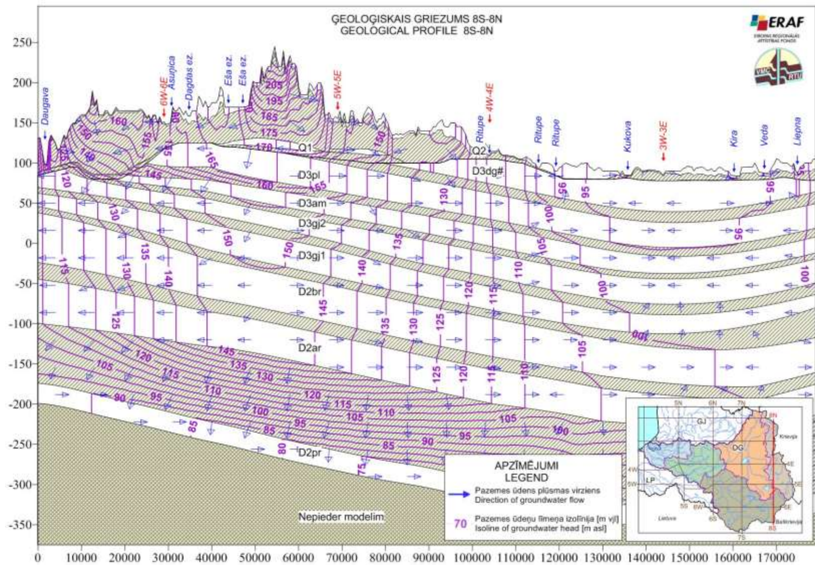
32. att. Ģeoloģiskais griezumš 8S-8N
