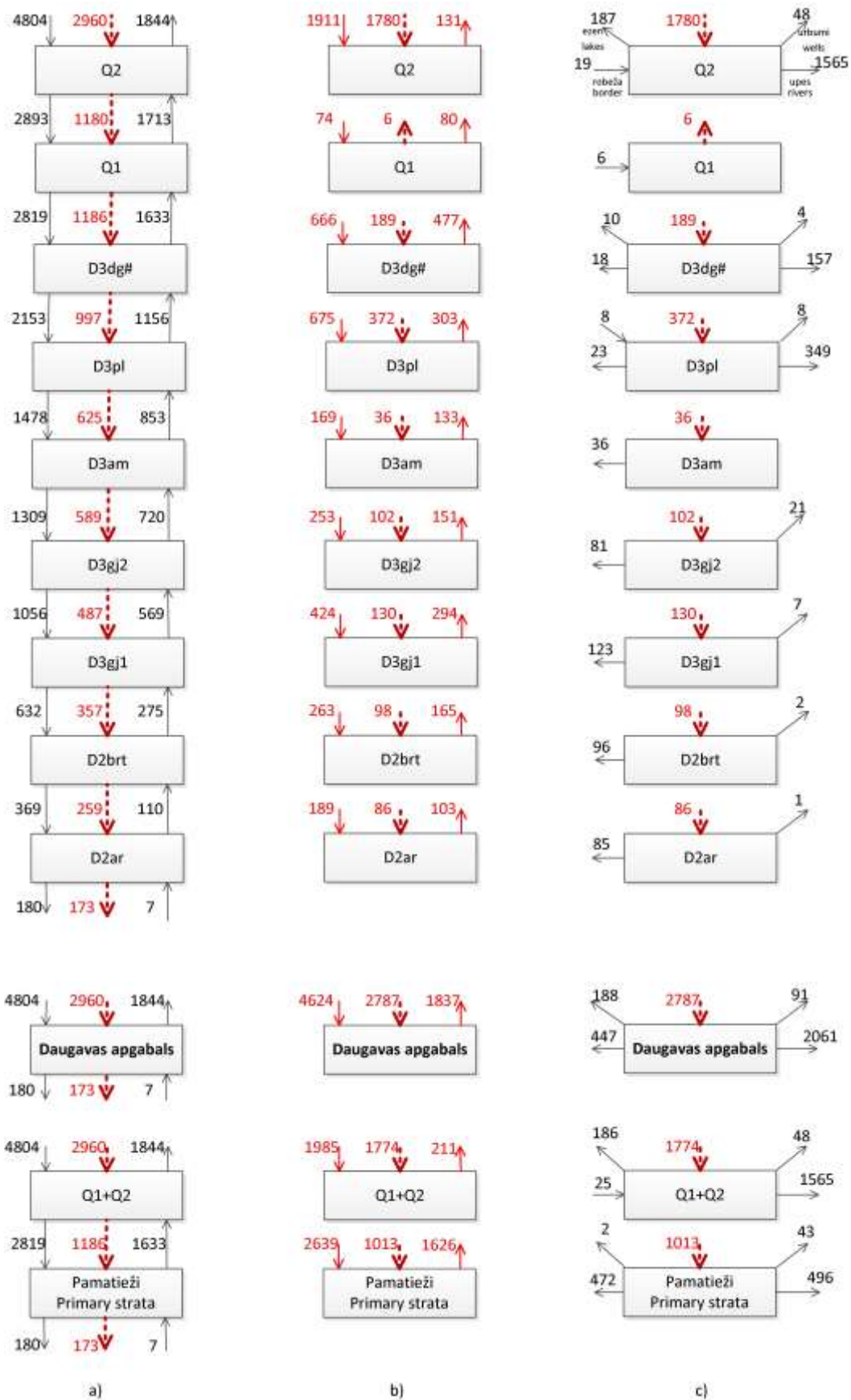
34. att. Pazemes ūdens balances [tūkst \text{m}^3/\text{dienn} ] shēma Daugavas apgabalā (grafiskais skaidrojums 2. tabulai)
