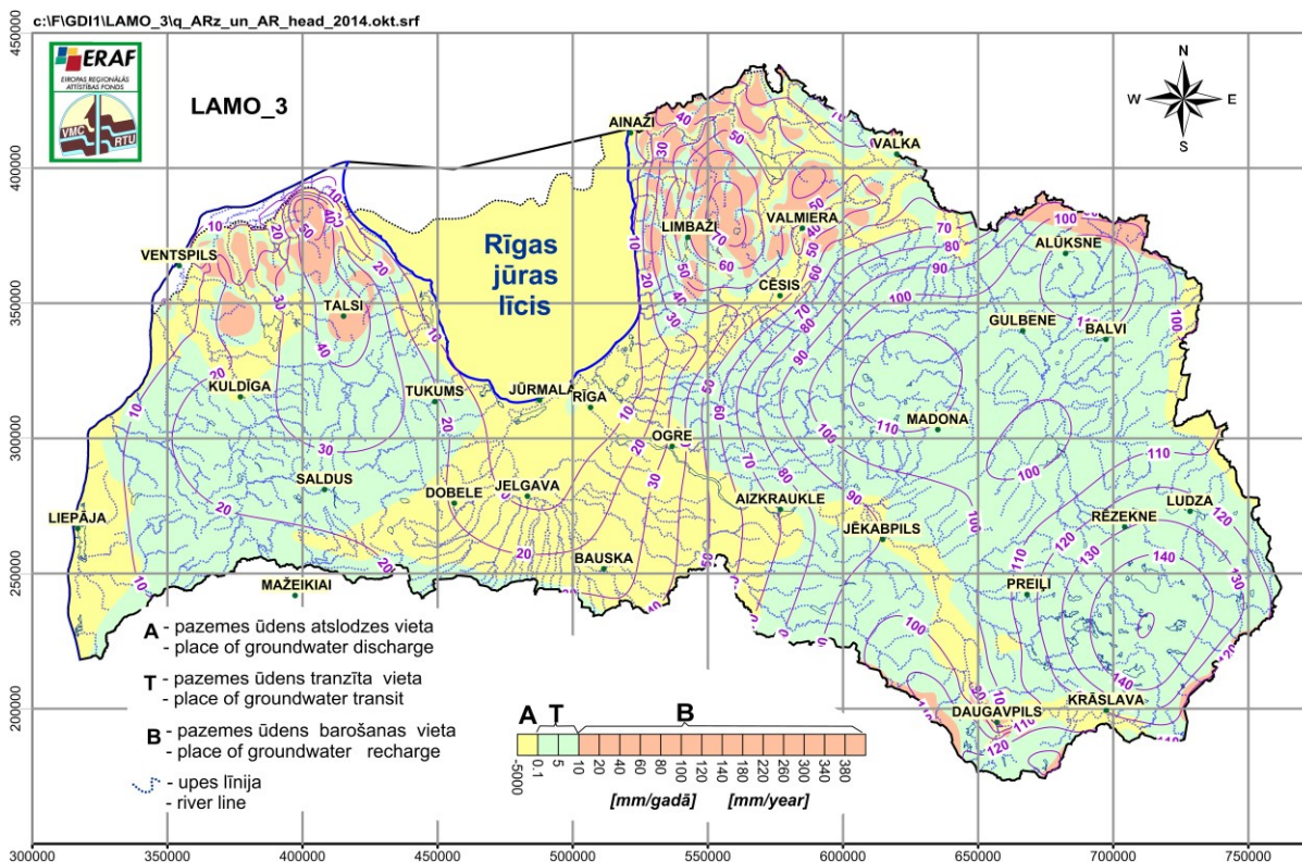
4. att. Plūsmu un ūdens līmeņu sadalījums D2ar horizontā LAMO2 un LAMO3
