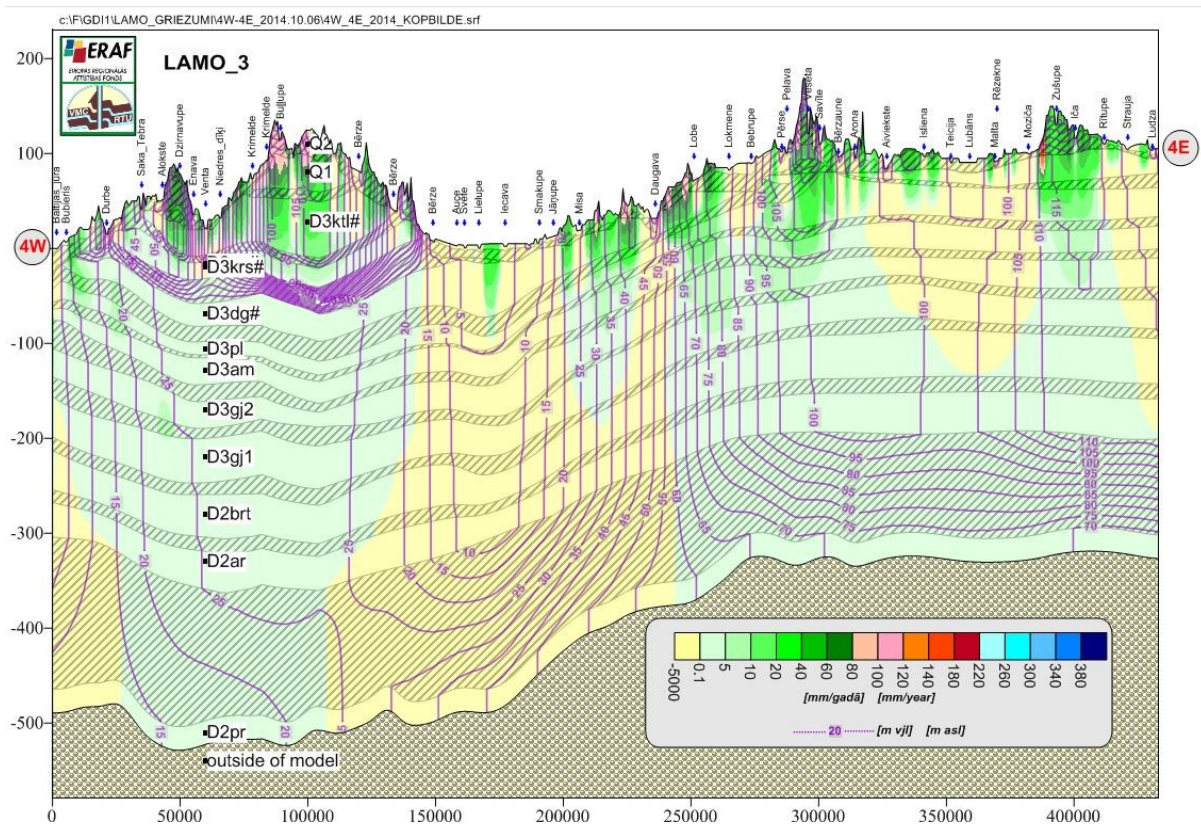
6. att. Ģeoloģiskais griezumš 4W-4E LAMO2 un LAMO3 versijās
