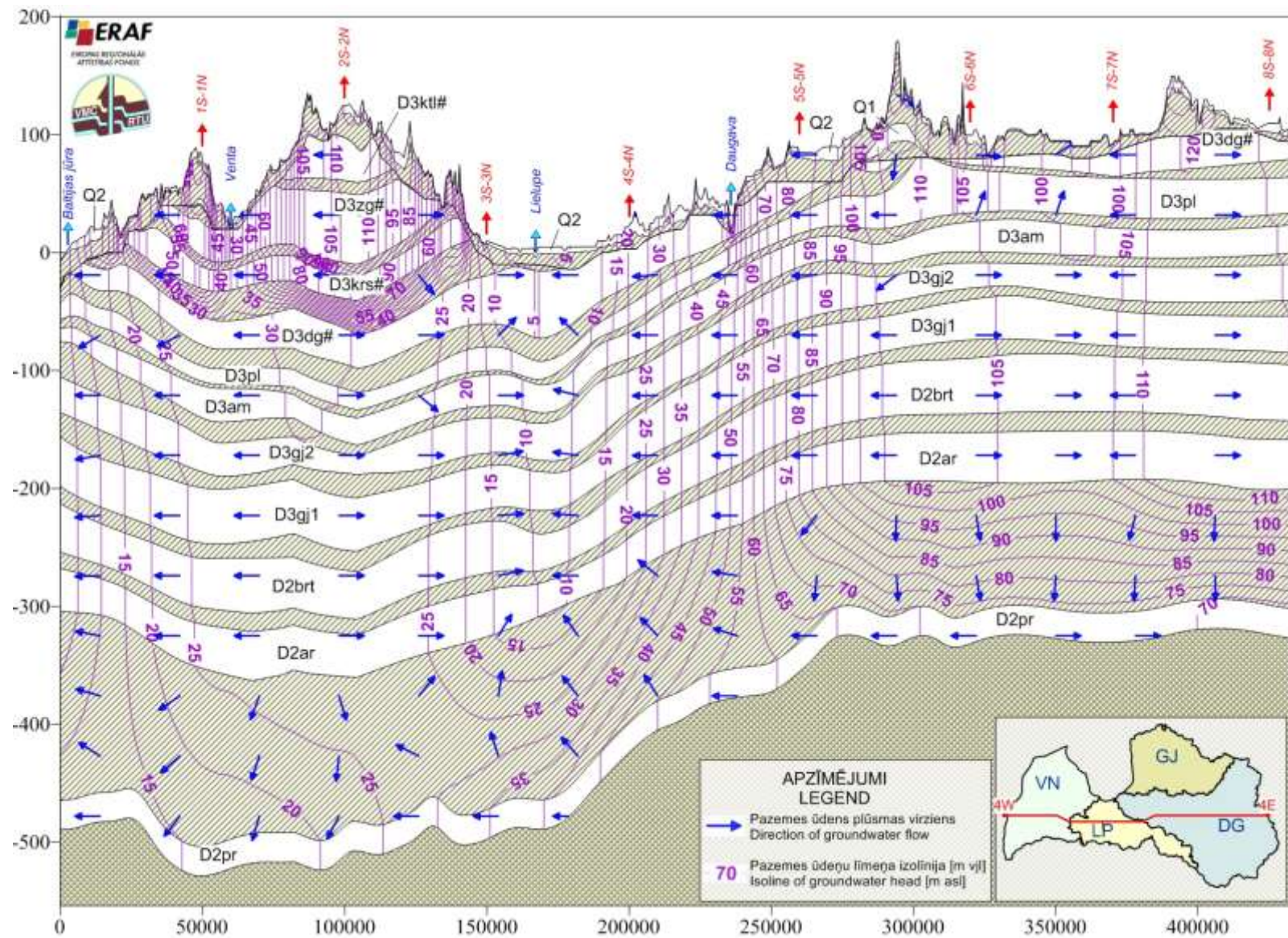
14p. att. Ģeoloģiskais griezumš 4W-4E
