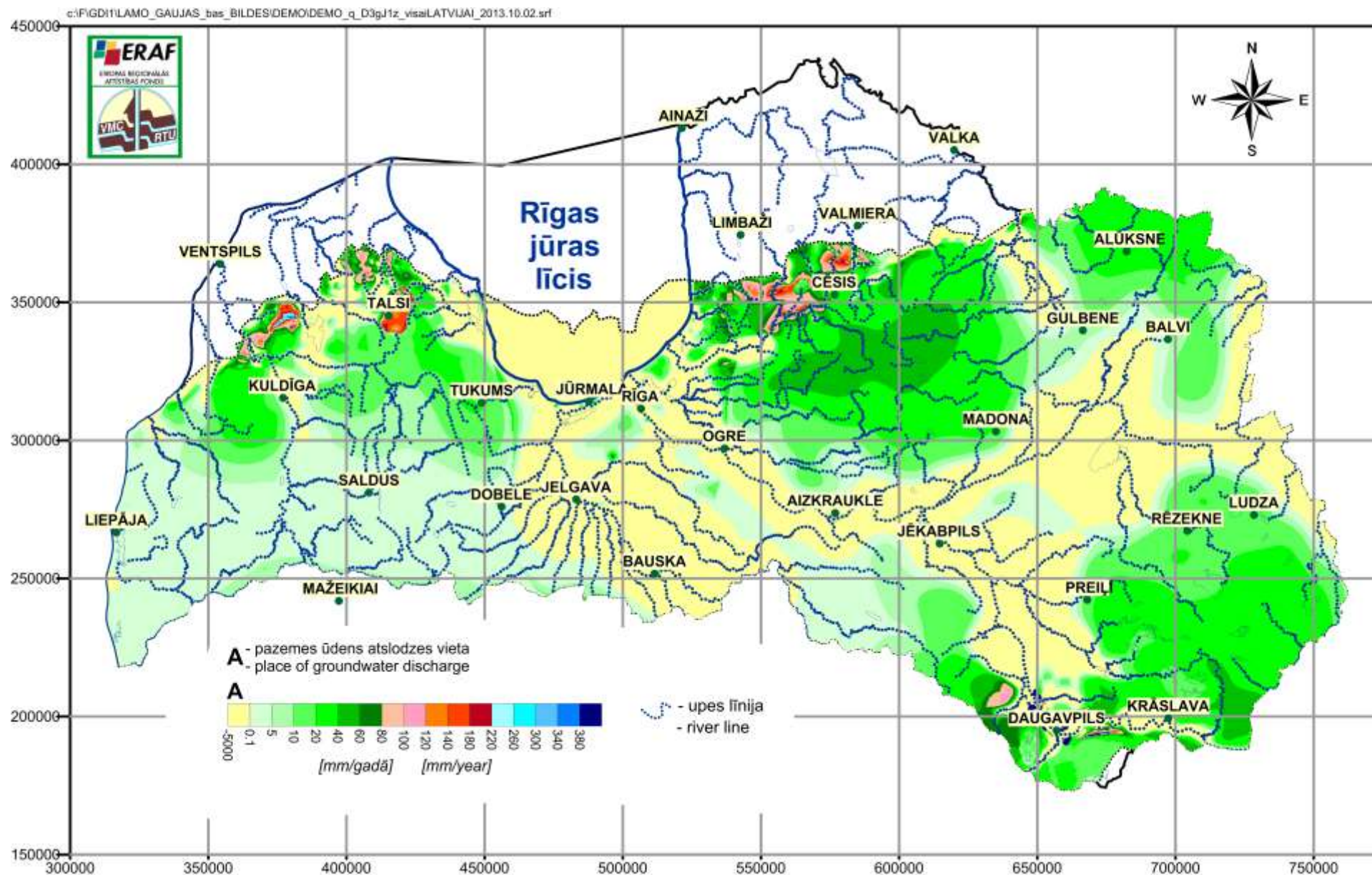
10p. att. Infiltrācijas plūsma D3gj1 horizontā [mm/gadā]
