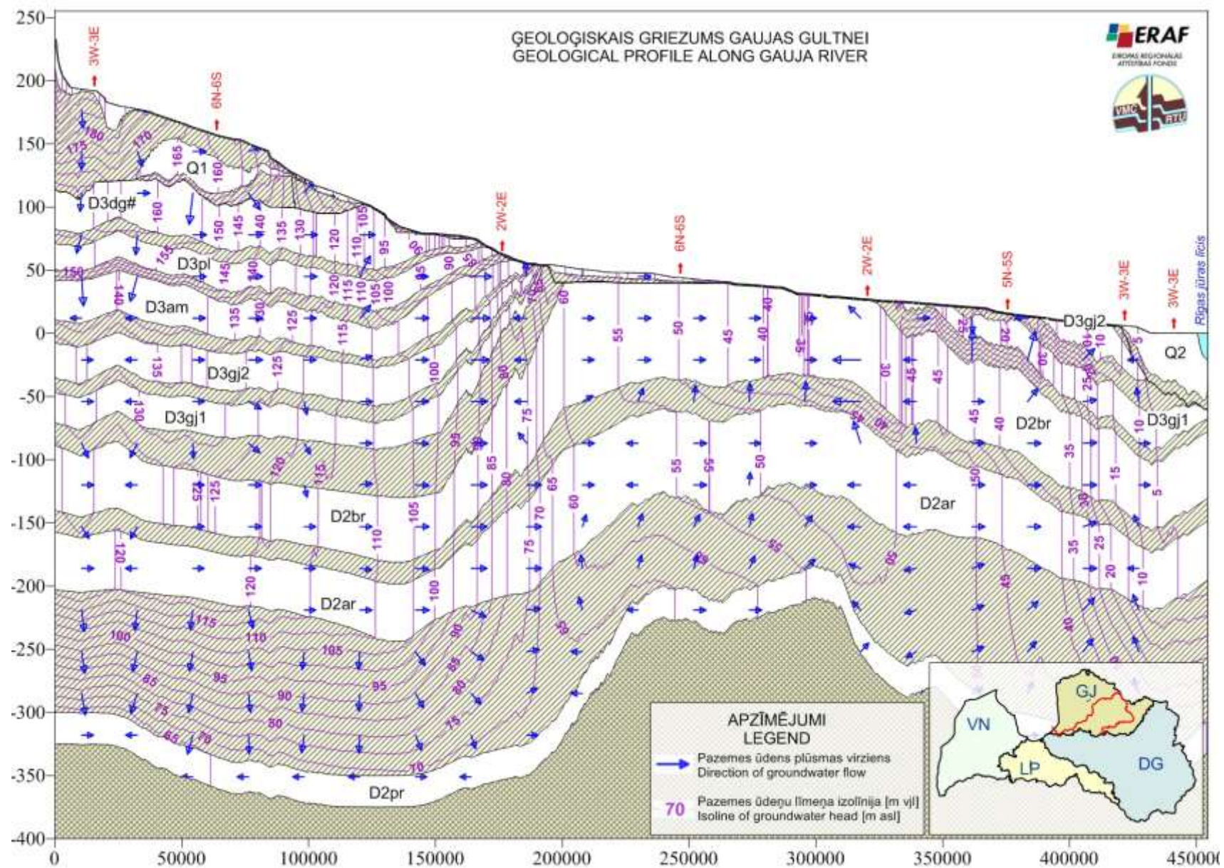
15p. att. Ģeoloģiskais griezumā pa Gaujas upi
