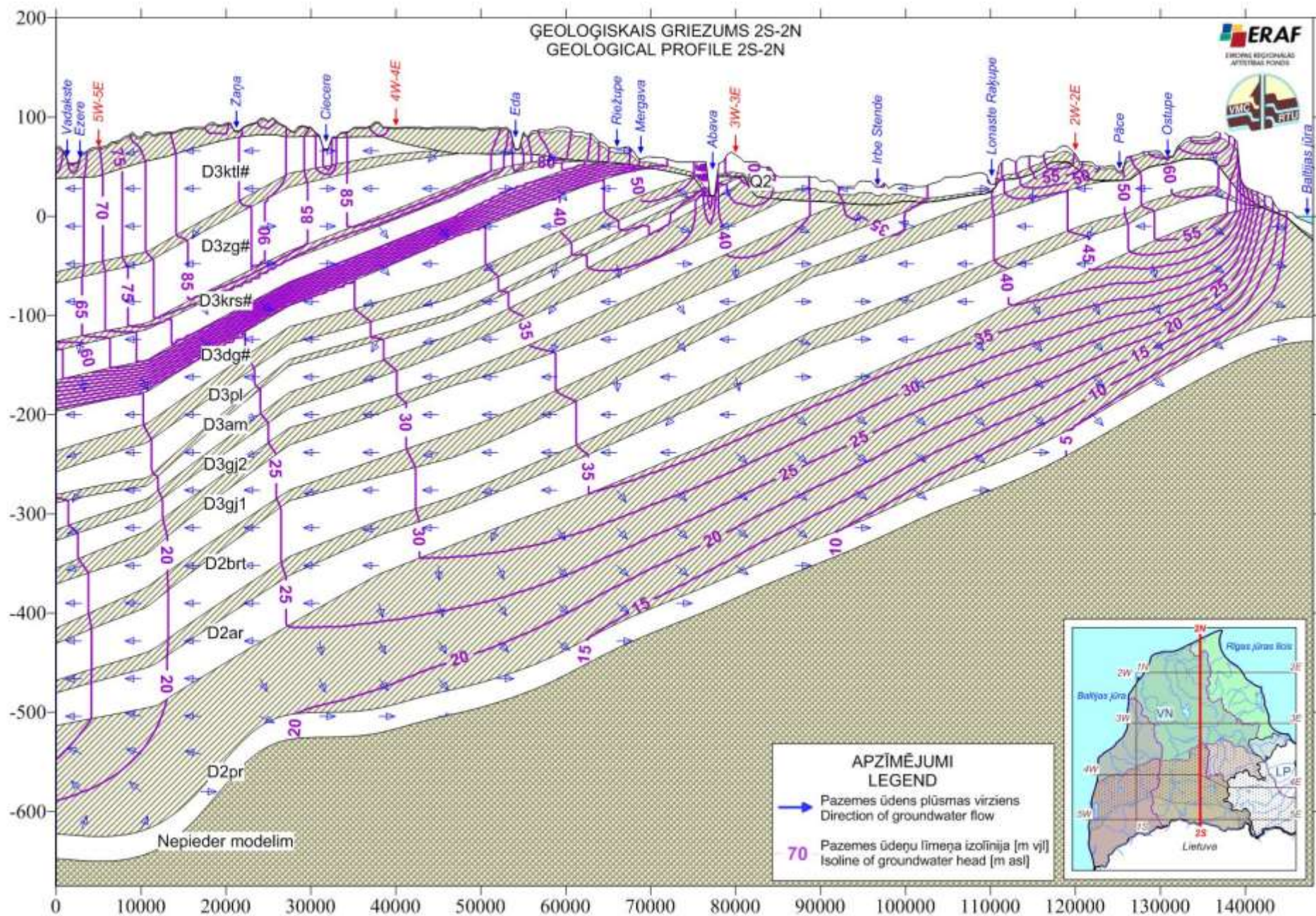
37. att. Ģeoloģiskais griezumums 2S-2N
