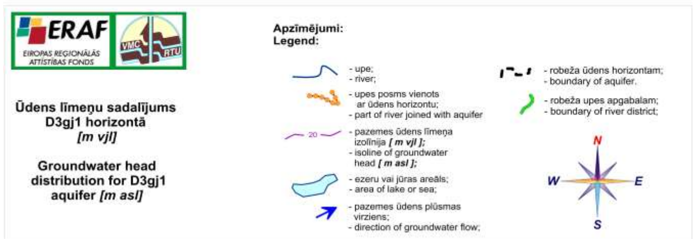
12. att. Ūdens līmeņu sadalījums horizontā D3gj1 [m vjl]
