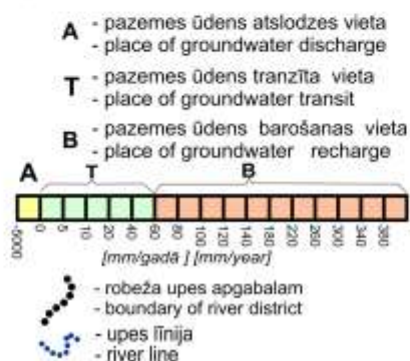
30. att. Pazemes ūdens plūsmas pamatiežu horizontā preQ
