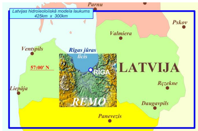
1. att. Reģionālo hidroģeoloģisko modeļu izvietojums
