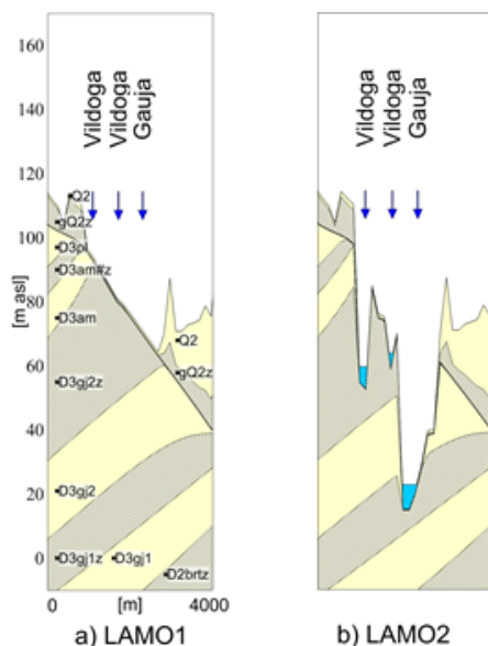
4. att. Gaujas un tās pieteces Vildogas ieleju iegrauzumi: a) LAMO1 – tikai Kvarāra slānī; b) LAMO2 – arī pamatiežos
