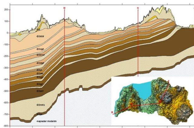
2. att. Ģeoloģiskais griezum
