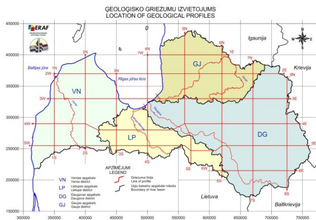
6. att. Latvijas upju lielbaseini un reģionālo ģeoloģisko griezumų izvietojums
