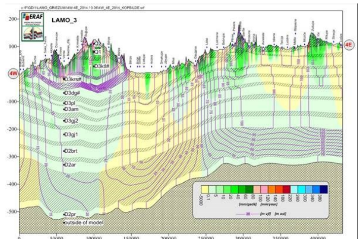
9. att. Ģeoloģiskais griezum 4W-4E LAMO3versijā
