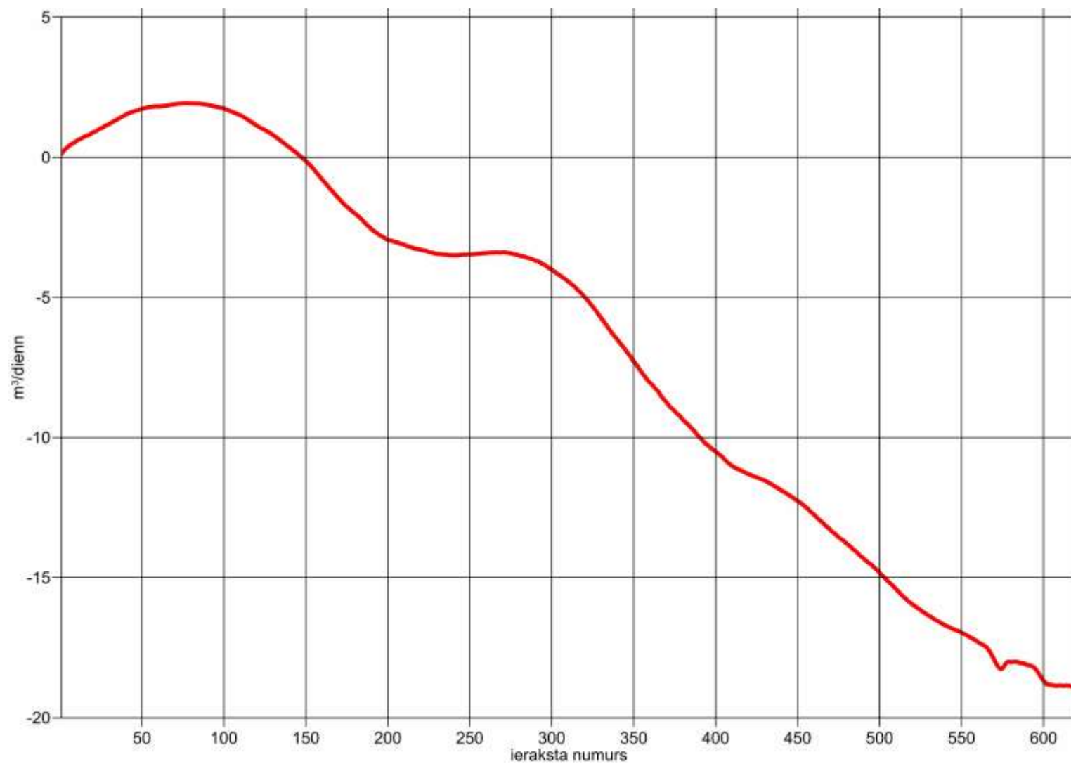
21. att. Uzpludinātā regulējamā grāvja pazemes ūdens pietece [ \text{m}^3/\text{dnn} ] lokālajā HM
