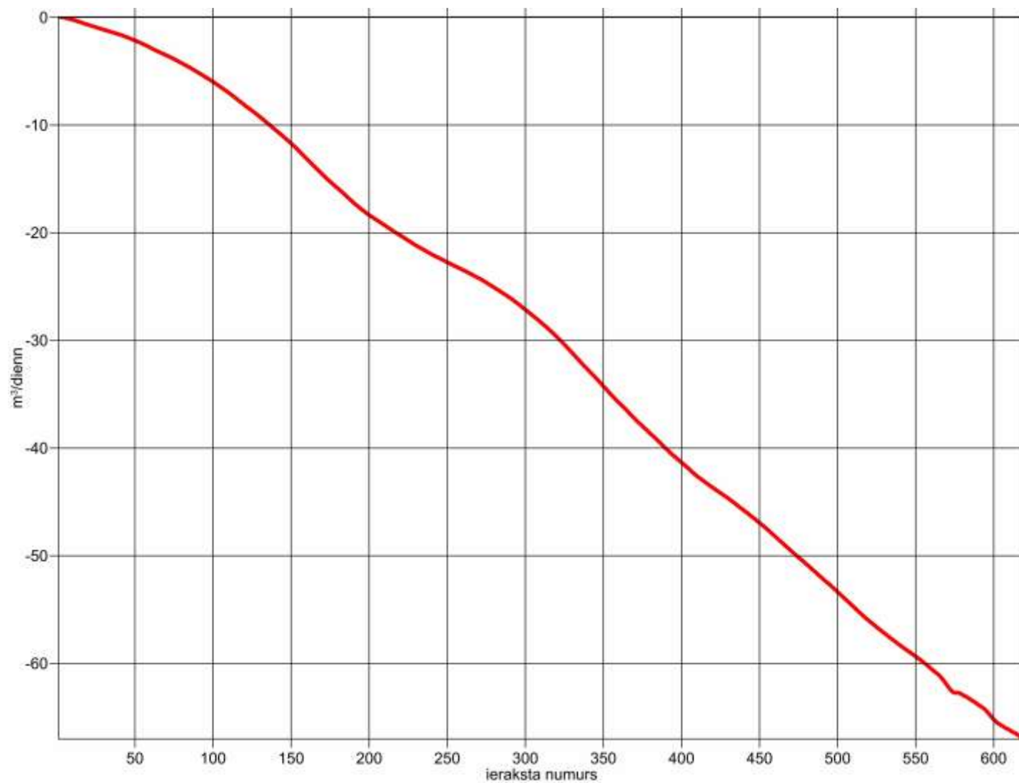
20. att. Regulējamā grāvja pazemes ūdens pietece [m³/dnn] lokālajā HM
